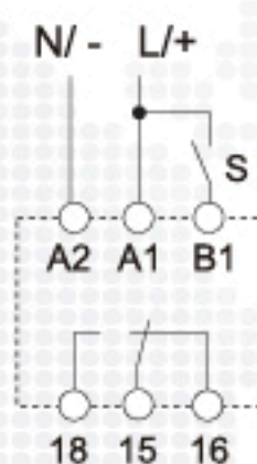
Esquema de conexión (con señal de mando)
