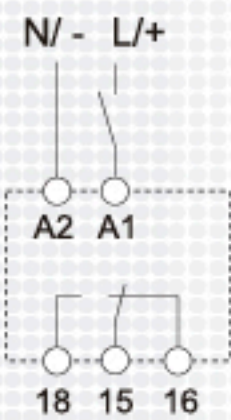
Esquema de conexión (sin señal de mando)
