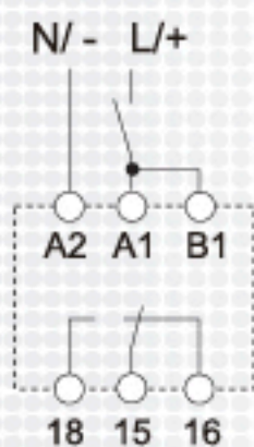
Esquema de conexión (sin señal de mando)
