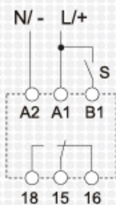
Esquema de conexión (con señal de mando)
